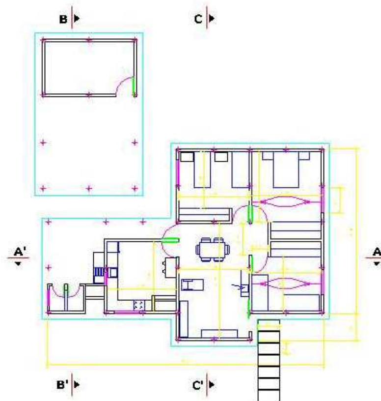
PLANTA DE DISTRIBUCIÓN
