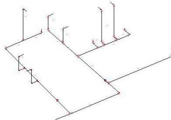
ISOMETRIA DE AGUAS BLANCAS
