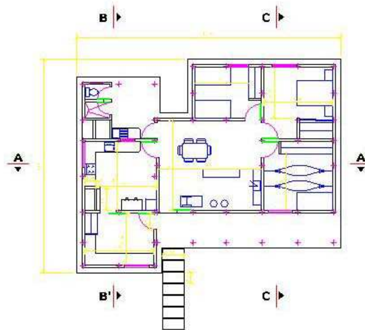
PLANTA DE DISTRIBUCIÓN
