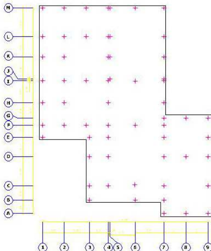
PLANTA DE ESTRUCTURAS
