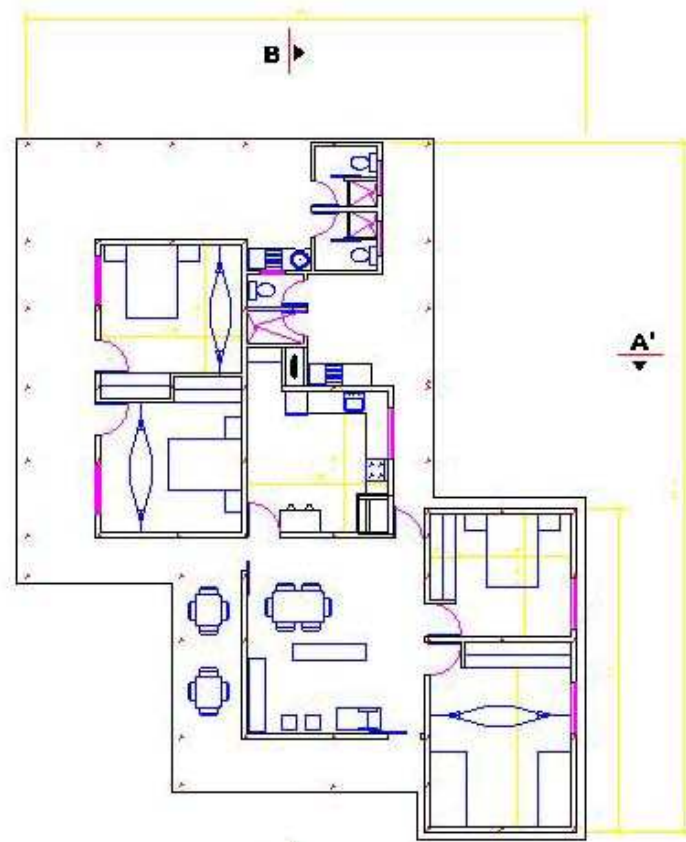
PLANTA DE DISTRIBUCIÓN
