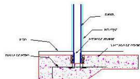
DETALLE DE UNION LOSA Y PANEL
