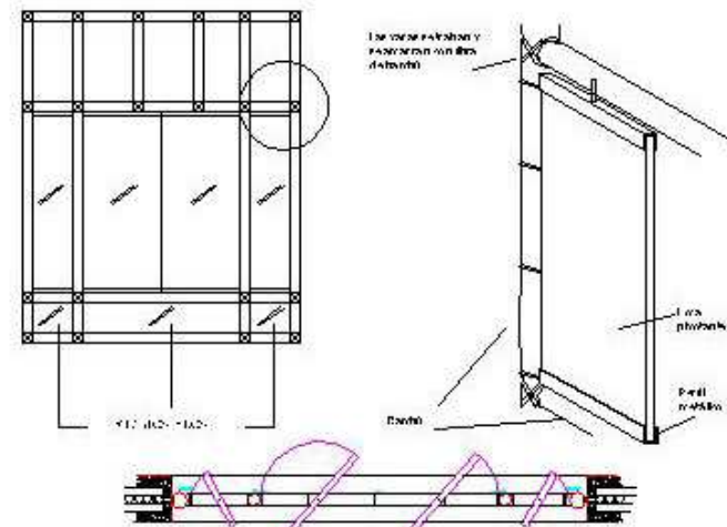
DETALLE DE LAS VENTANAS
