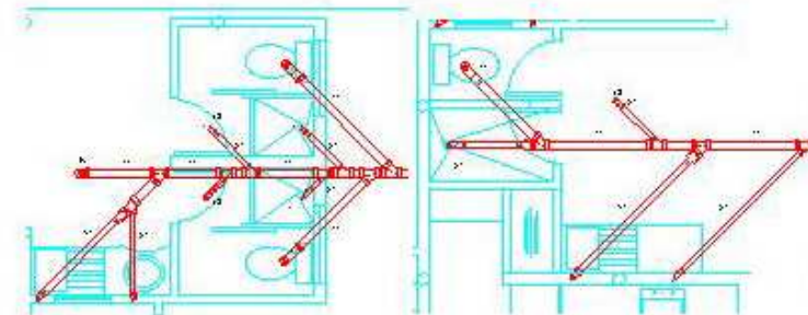
DETALLE DE AGUAS NEGRAS
